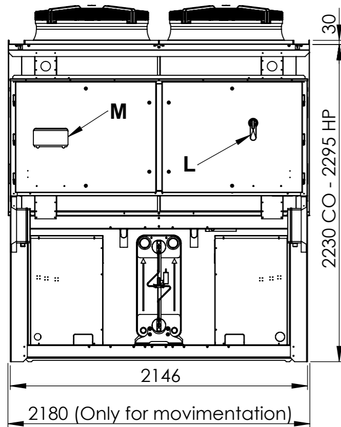
VISTA FRONTALE TOP VIEW
