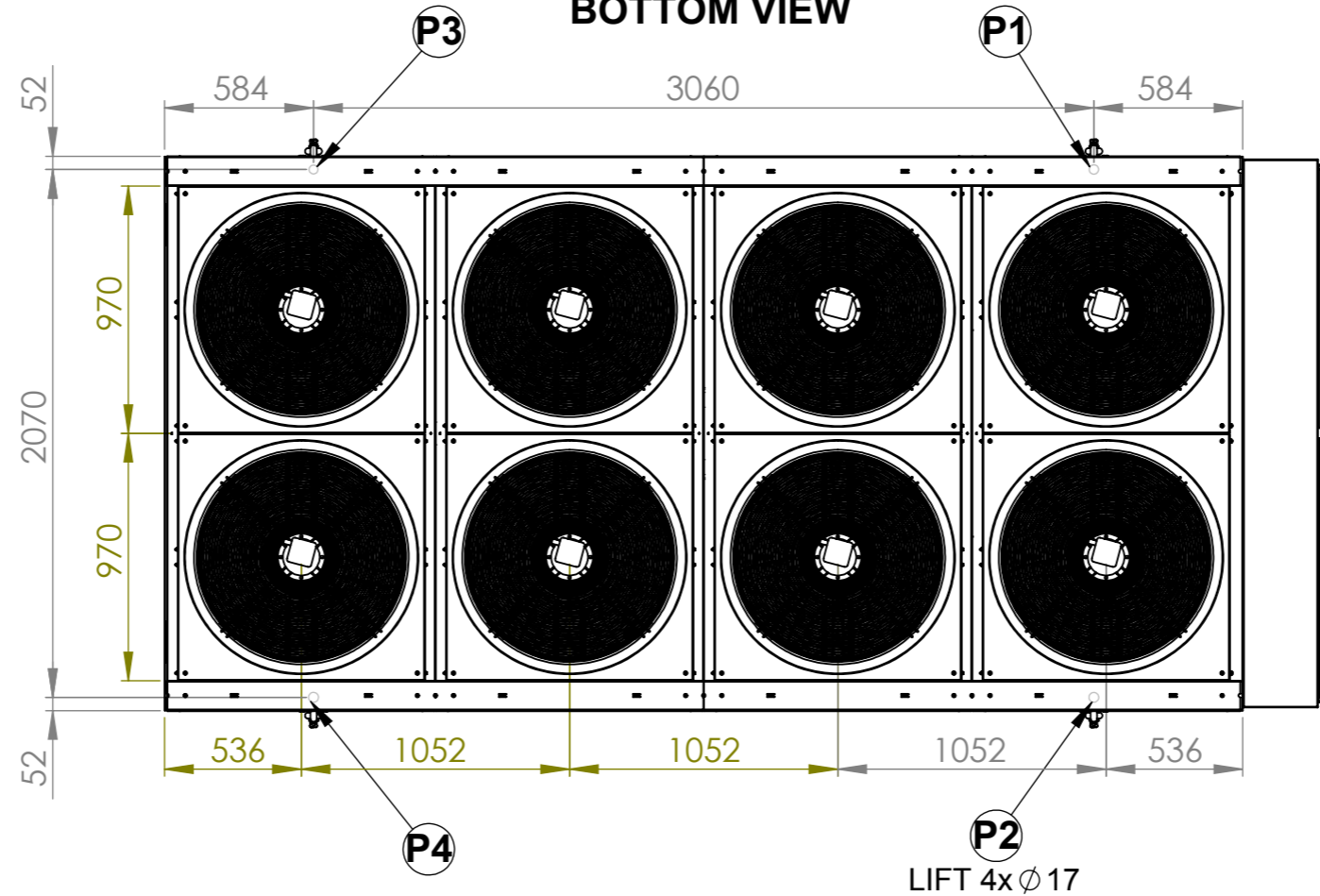
VISTA DALL'ALTO BOTTOM VIEW
